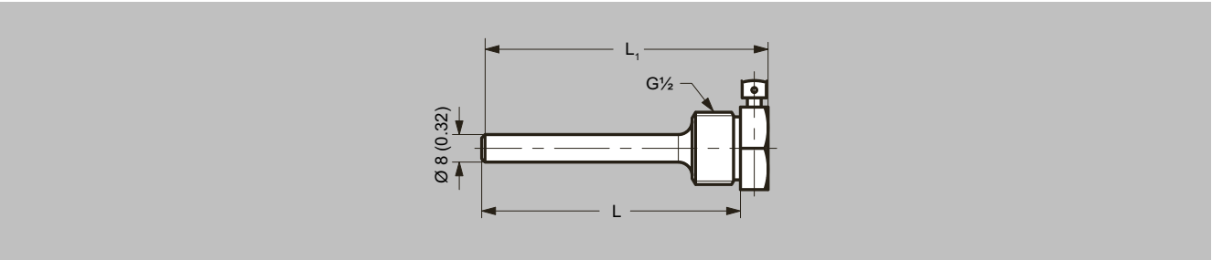
Vaina de sensores, latón (solo para los Pt500 a 2 hilos), dimensiones en mm (pulgadas)
