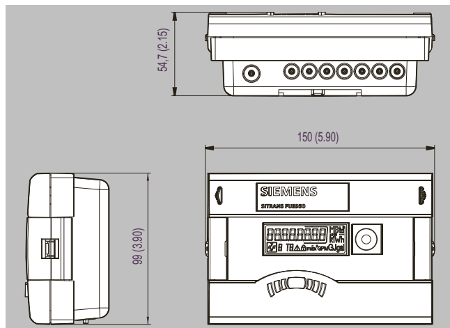
SITRANS FUE950, dimensiones en mm (pulgadas)
